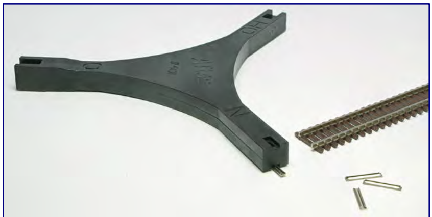
Mit diesem Hilfswerkzeug (Art.-Nr. 401) werden die von der Spur N stammenden Schienenverbinder (2090) verletzungsfrei aufgesetzt.
