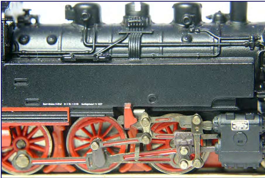
Allen Unkenrufen zum Trotz ist die Nachbildung des Gestänges hervorragend gelungen. Erstmals hat Märklin auch den Fangbügel für die Treibstange nachgebildet (zu sehen zwischen 1. Kuppel- und der Treibachse) Auch der Dampfzylinder zeigt sich sehr detailliert und mit einer Nachbildung des Fabrikschildes.
